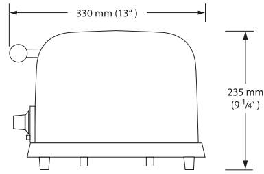
側視圖
