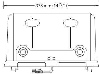
正視圖
