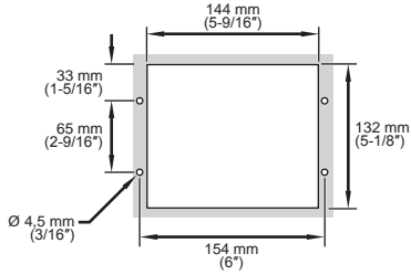
RCTHW-1B 控制盒开口尺寸
