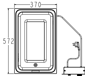
顶视图
