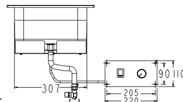
正视图
