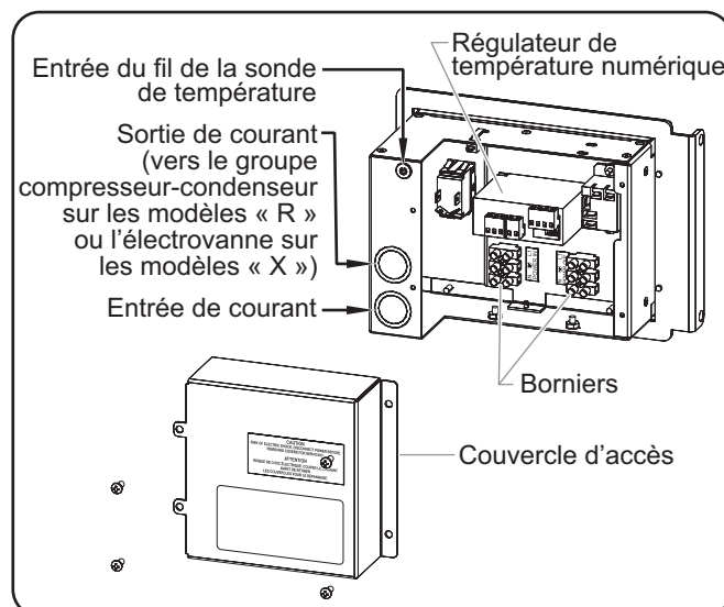
Raccordements du système réfrigéré contrôlé à distance
