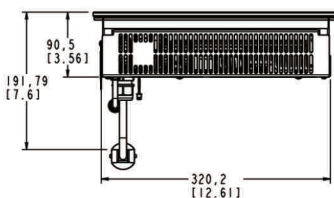
侧视图
