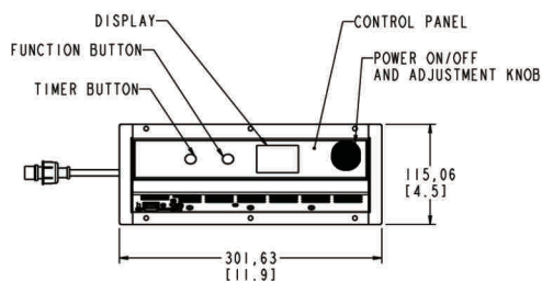
正视图
