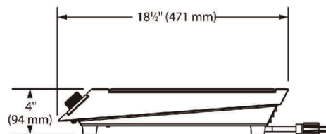
侧视图
