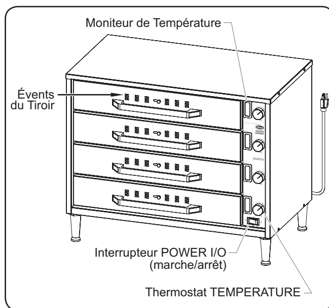
Modèle HDW-2R2
