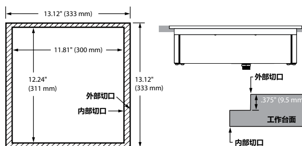
正视图
