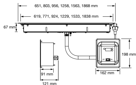
侧视图
