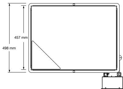
顶视图
