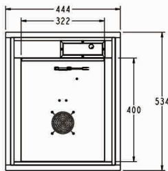
正视图
