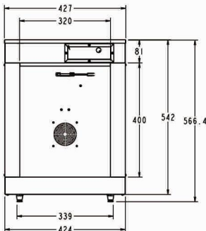
正视图
