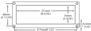
控制盒开孔尺寸
