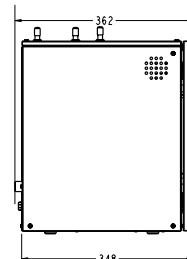
水箱侧视图
